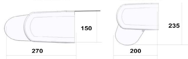
Montaż ścienny
