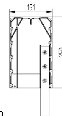
VBox ECO doppelseitiger Träger
