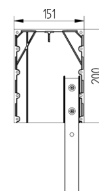
VBox ECO doppelseitiger Träger
