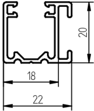
Führungsschiene Typ 2
