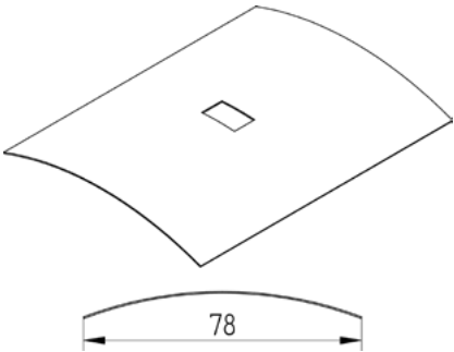
Querschnitt von C-80 Flachlamellen
