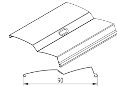
Querschnitt von Z-90-Lamellen
