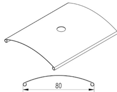
Querschnitt von C-80-Lamellen
