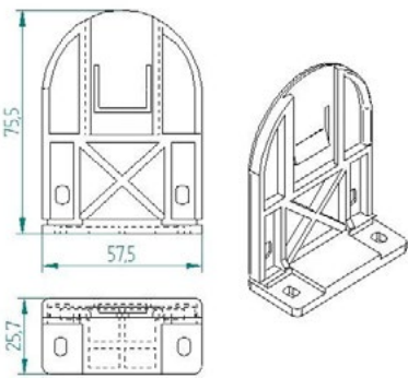
PVC Hänger
