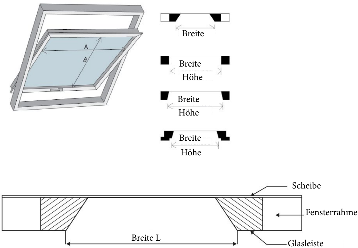
Breite und Höhe von Dachfensterrollos - Abstand zwischen Glasleistenränden
