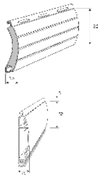
LDG/52
