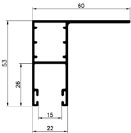
PK 53
