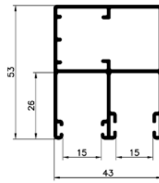
PP 53/ODS
