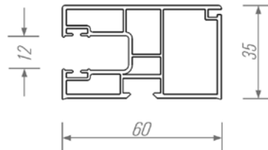
PG 01
