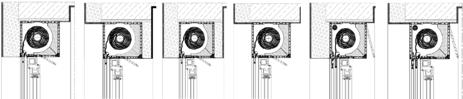
Typ „A“
