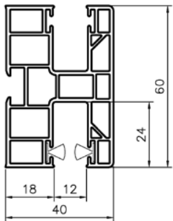
PPD 60/12
