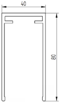
Top priofile
