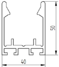
Side door frame
