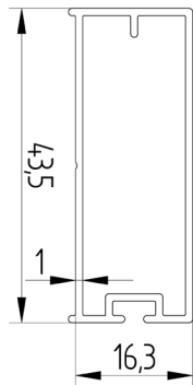
Plisse 20 mm side door frame profile
