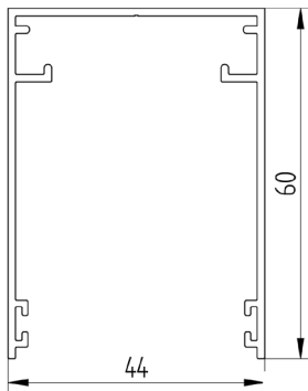
Plisse 20 mm top door frame profile
