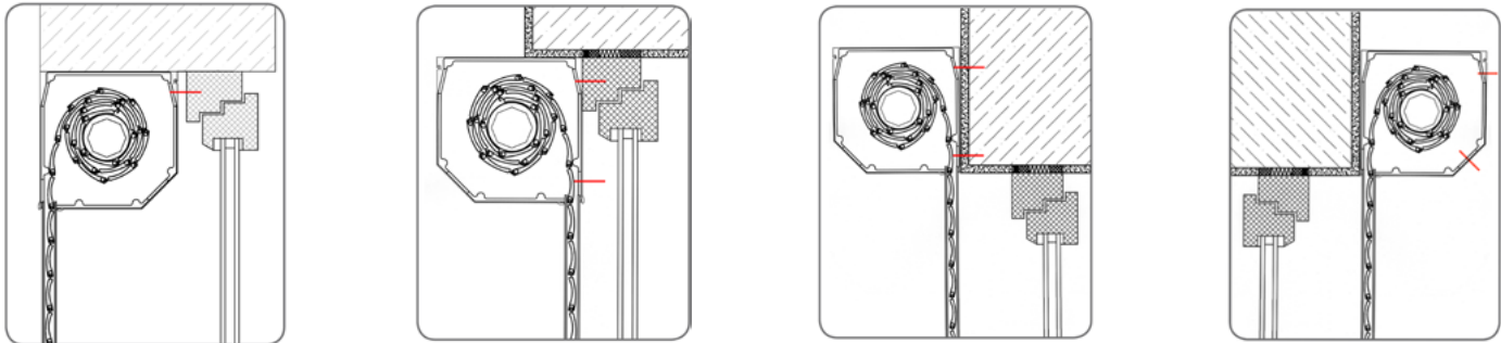
Typ „A“ IN DER FENSTERNISCHE (RECHTSROLLER).
