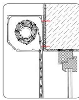
Typ „C“ Linksroller auf Mauerwerk
