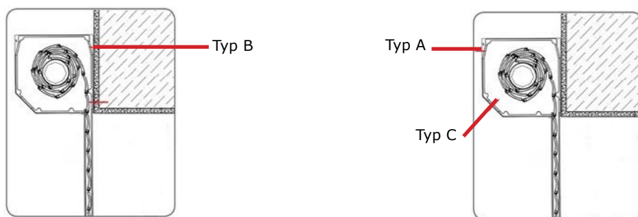
Typ A - Kardangelenk 90 Grad Typ B - Kardangelenk 90 Grad Typ C - Kardangelenk 45 Grad
