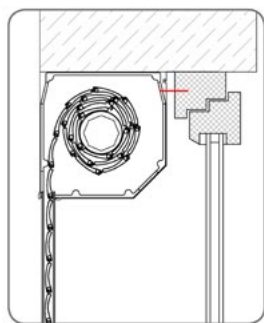
Typ „A“ Rechtsroller
