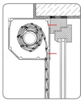
Typ „B“ Linksroller in der Leibung
