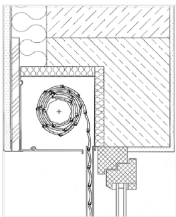
Rolladenkasten eingebaut während Mauerbau
