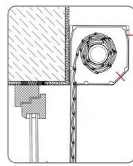
Typ „D“ Rechtsroller auf Mauerwerk
