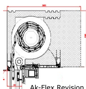
Ak-Flex Revision von Innen
