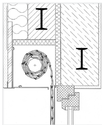
Rolladenkasten eingebaut in Wandsturz
