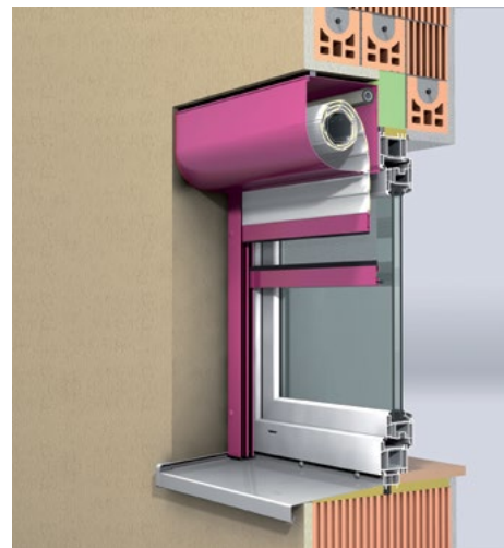
SKRZYŃKA ĆWIERĆOKRĄGŁA
