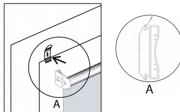
5. Wkliknąć profil nośny w klipy.
