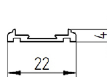
Schwelle 4 mm
