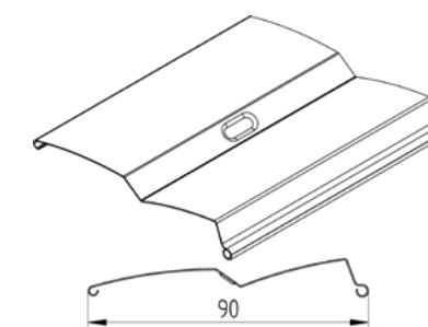
Lamellenquerschnitt Z-90
