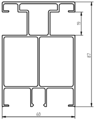
Führungsschiene PG-10
