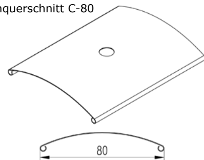
Lamellenquerschnitt C-80
