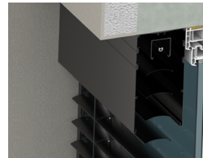
Montage in der Leibung
