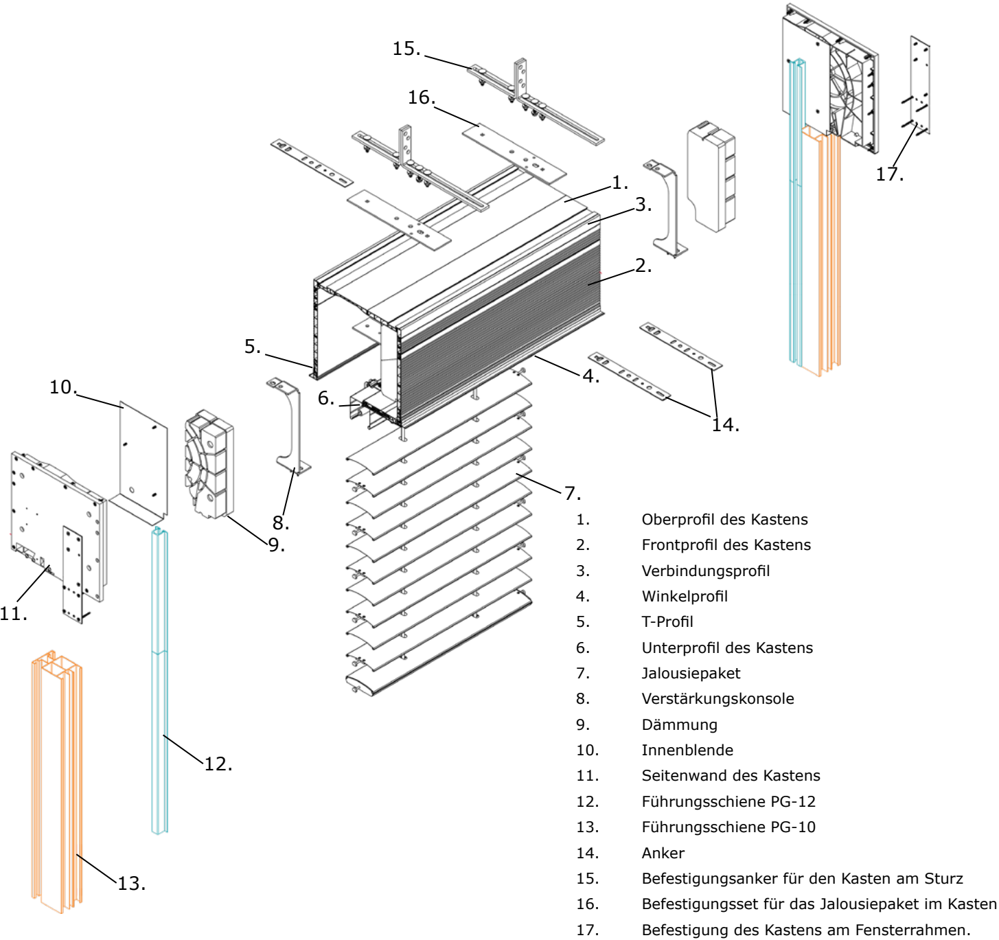
Führungsschiene PG-10
