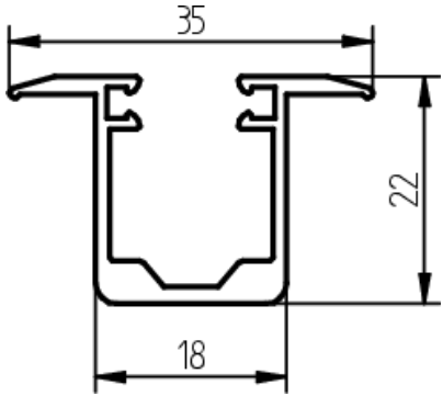
Führungsschiene PG-12
