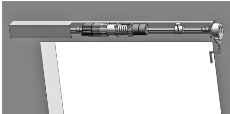
Schema der Außenjalousie mit NHK-System
