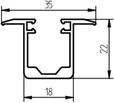
Prowadnica PG-12
