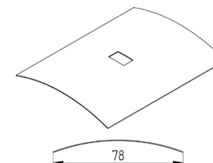
Przekrój lameli C-80 Flat
