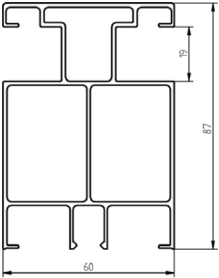
Prowadnica PG-10
