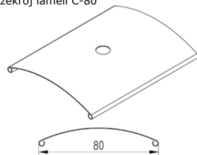
Przekrój lameli C-80
