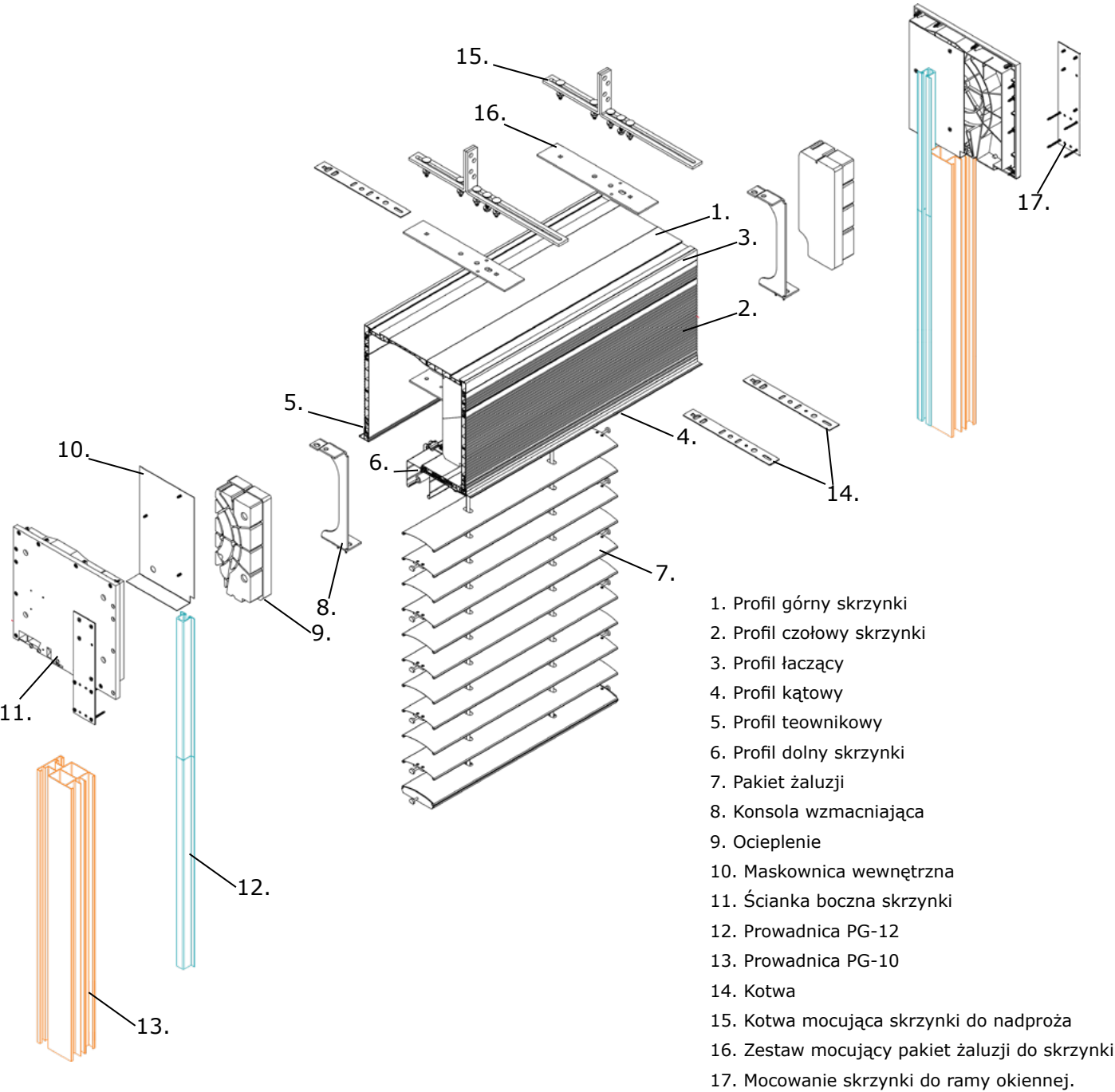
Prowadnica PG-10
