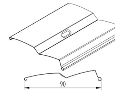
Przekrój lameli Z-90
