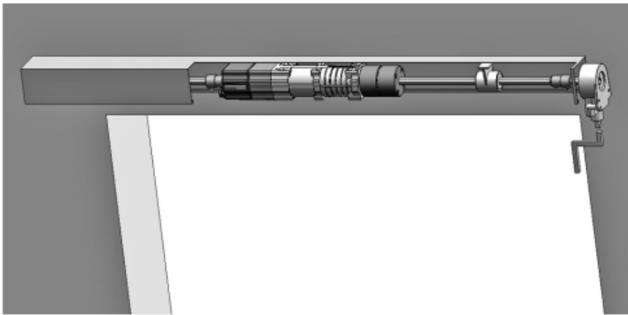
Schemat żaluzji fasadowej z sytemem NHK
